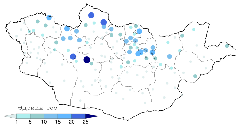
Зураг 4. -30^{\circ}\text{C} -аас хүйтэн өдрийн тооны оронзайн тархалт
