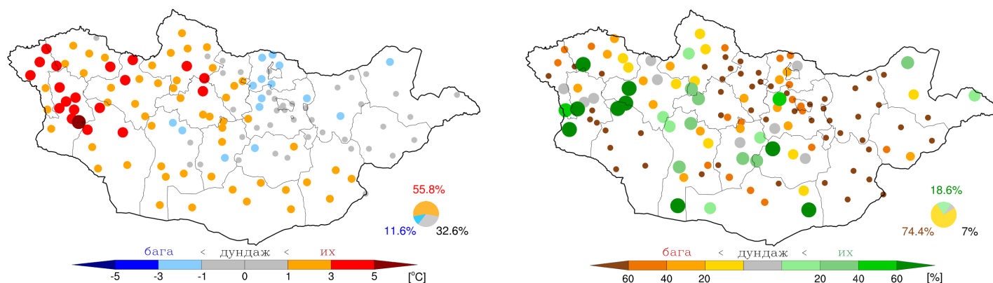
Зураг 2. 2025 оны 12 дугаар сарын агаарын дундаж температур, нийлбэр хур тунадасны ОЖД-аас хазайх хазайлтын оронзайн тархалт
