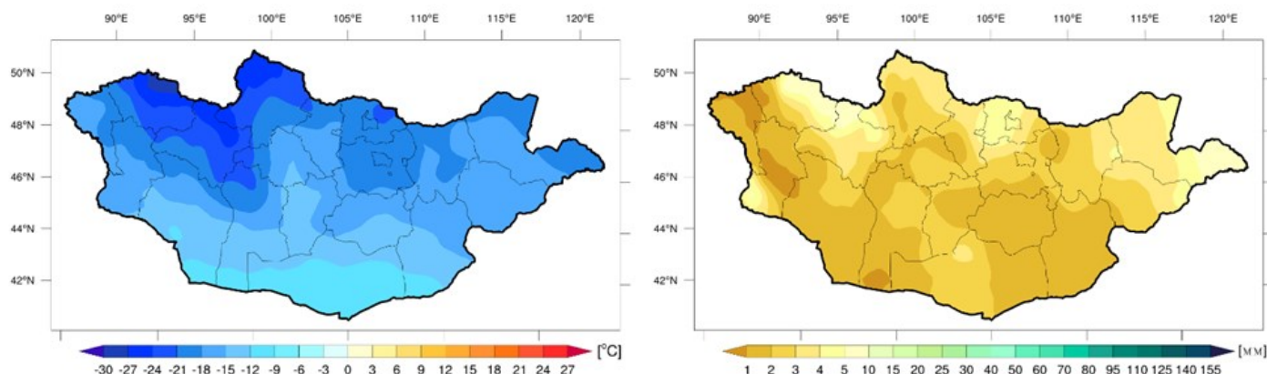
Зураг 1. 1991-2020 оны 12 дугаар сарын агаарын дундаж температур, нийлбэр хур тунадасны оронзайн тархалт
